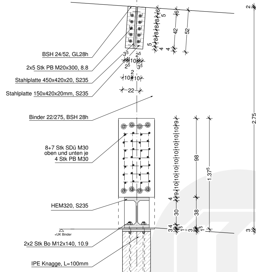
Seitenansicht Binder
