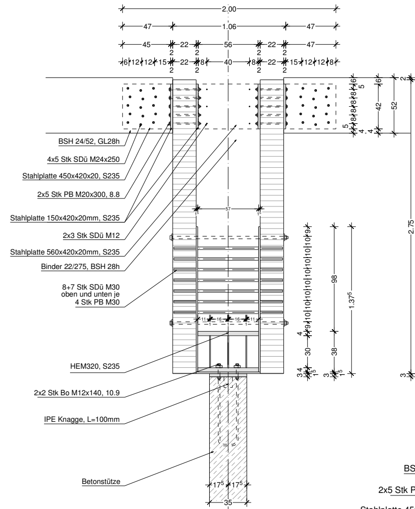
Vertikaler Schnitt Binder
