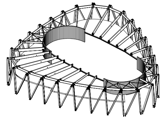
Isometrie Holzkonstruktion müllerblaustein
