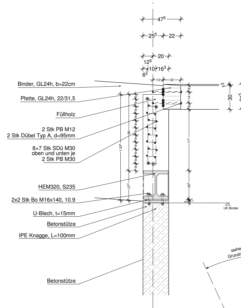
Vertikaler Schnitt Binder / Traufe
